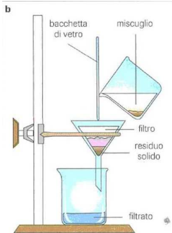
Schema filtrazione:
